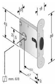
Edelstahl
